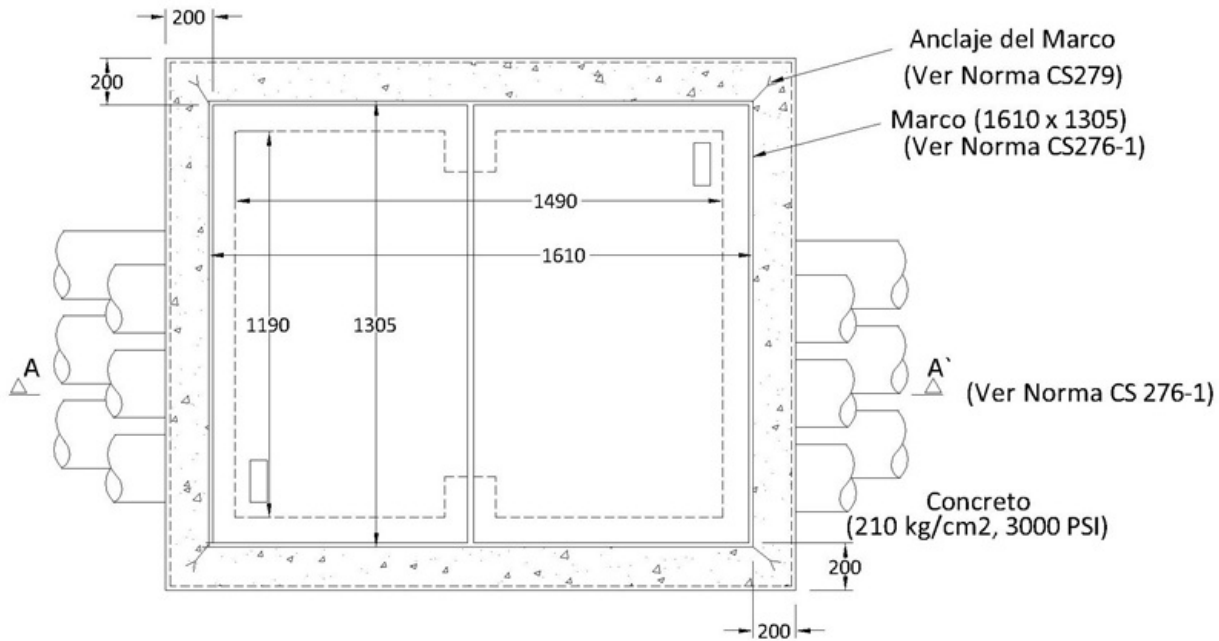
PLANTA CAJA DOBLE CON MARCO
