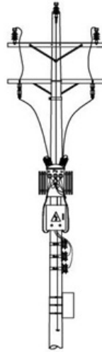
DISPOSICIÓN TRIANGULAR TRAFO BIFILAR CTR 505
