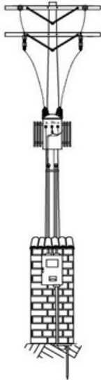
FINAL DE CIRCUITO BIFILAR TRAFO BIFILAR CON ACOMETIDA EN B.T CTR 505-1
