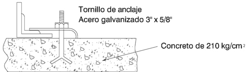
DETALLE PERNO DE ANCLAJE
