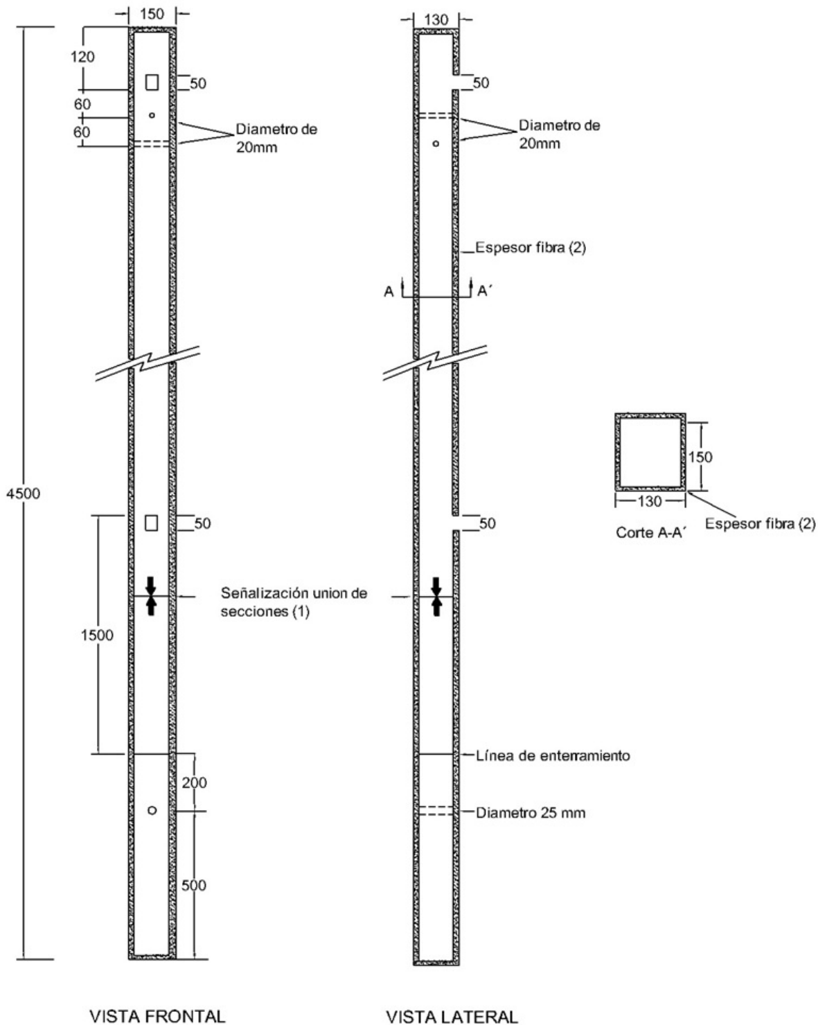
FIGURA 1. ESQUEMA POSTE EN FIBRA
