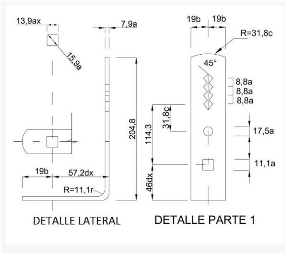
FIGURA 1- A: Soporte para fijación a cruzeta, detalle parte 1. Dimensiones en milímetros [mm]
