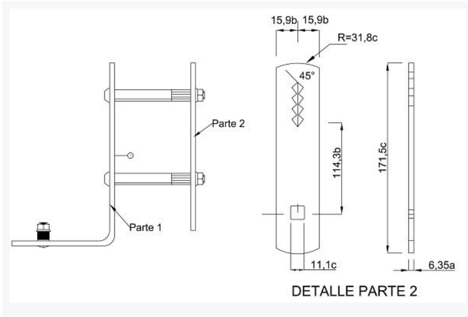
FIGURA 1-B: Soporte para fijación a cruzeta, detalle parte 2. Dimensiones en milímetros [mm]
