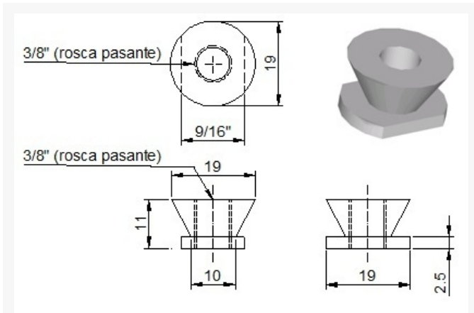
Figura 2. Tornillo pasante y tuerca
