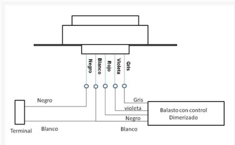
Figura 3 Diagrama de conexionado.
