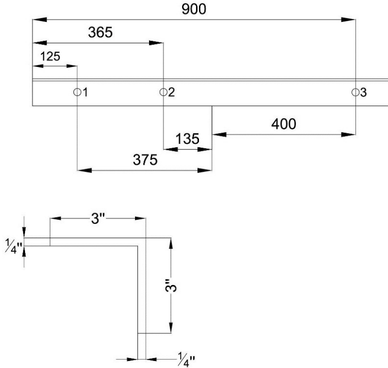
Figura 1. Cruceta Metálica de 1m
