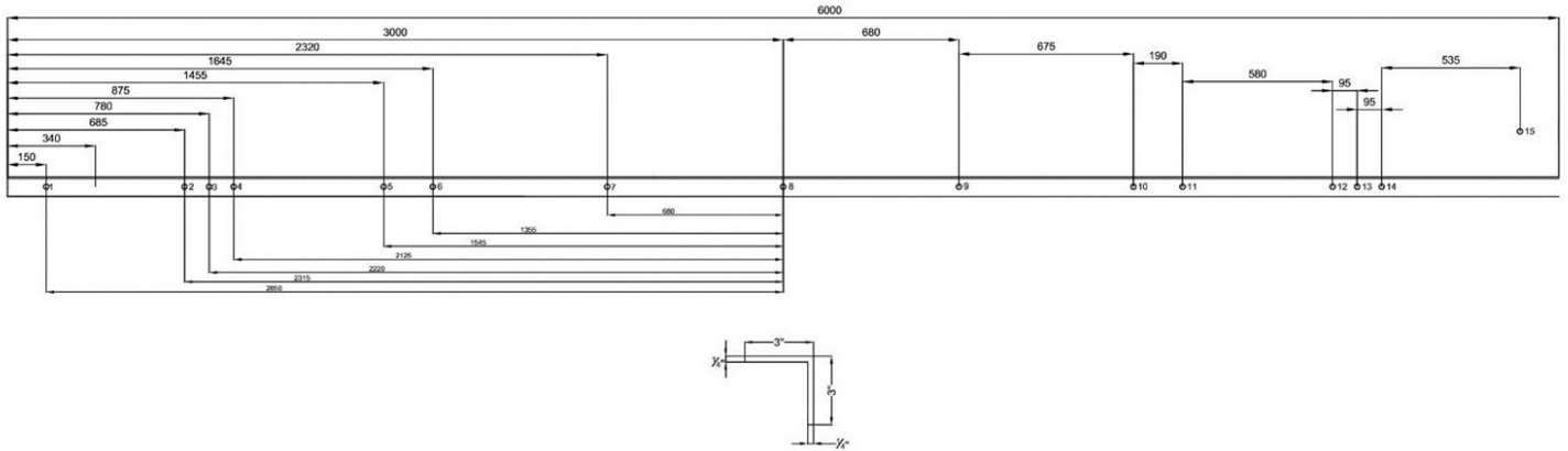
Figura 4. Cruceta metálica de 6m
