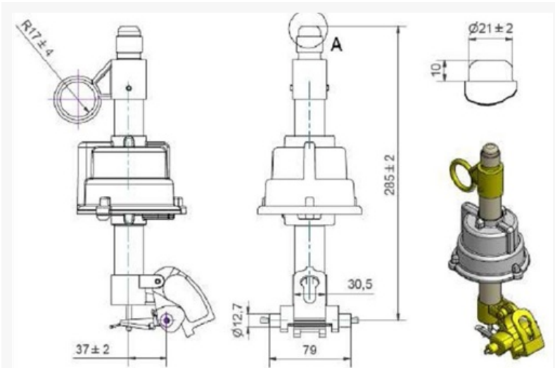
Figura 2. Dimensiones referenciales equipo 15 kV, en mm.
