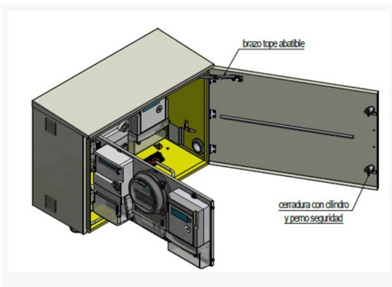
FIGURA 5. UBICACIÓN DE EQUIPOS
