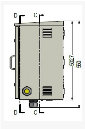
FIGURA 2. VISTA DE COSTADO
