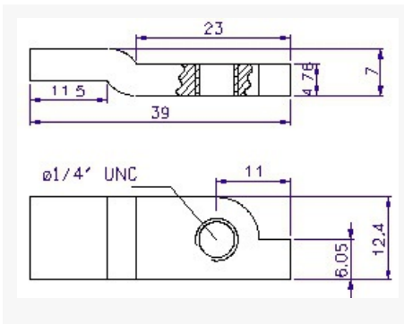
FIGURA 14: PLATINA DE CIERRE
