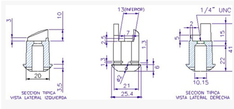
FIGURA 6: BUJE DEL SISTEMA DE SEGURIDAD
