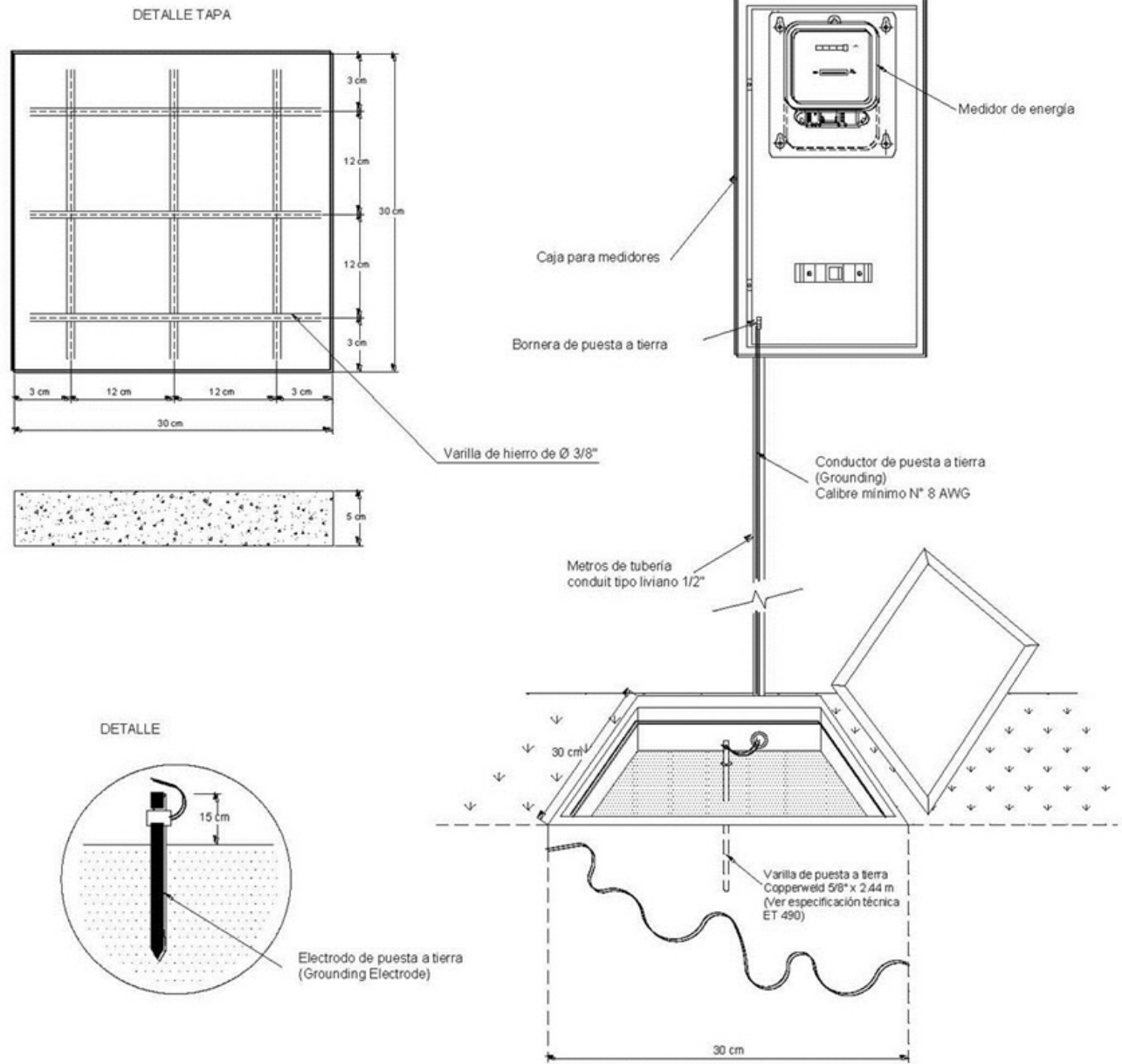
ELEMENTOS DE PUESTA A TIERRA EN BAJA TENSIÓN
