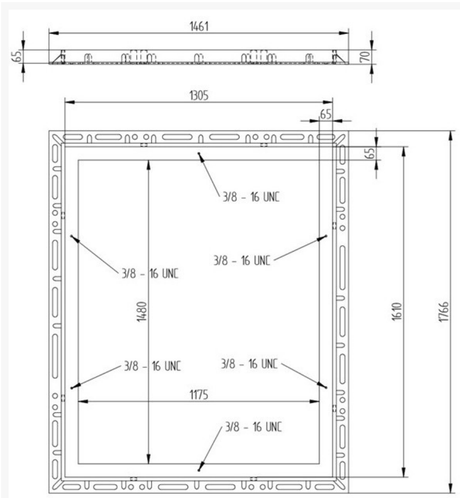
Fig. No. 5 Marco para caja de inspección doble de MT y BT
