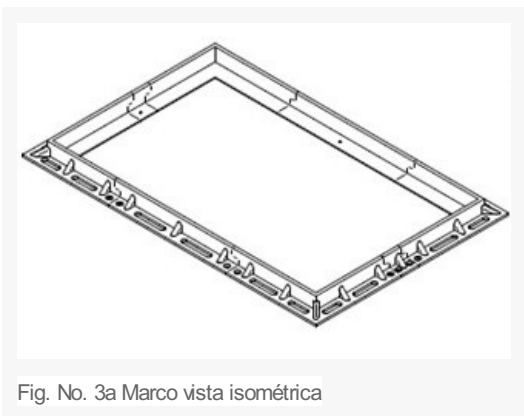
Fig. No. 3 Marco para caja de inspección sencilla de MT y BT
