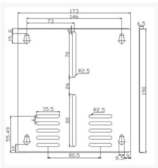
FIGURA 4: BANDEJA PARA MEDIDOR MONOFÁSICO
