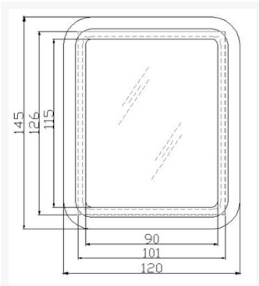
FIGURA 5: VENTANA DE INSPECCIÓN
