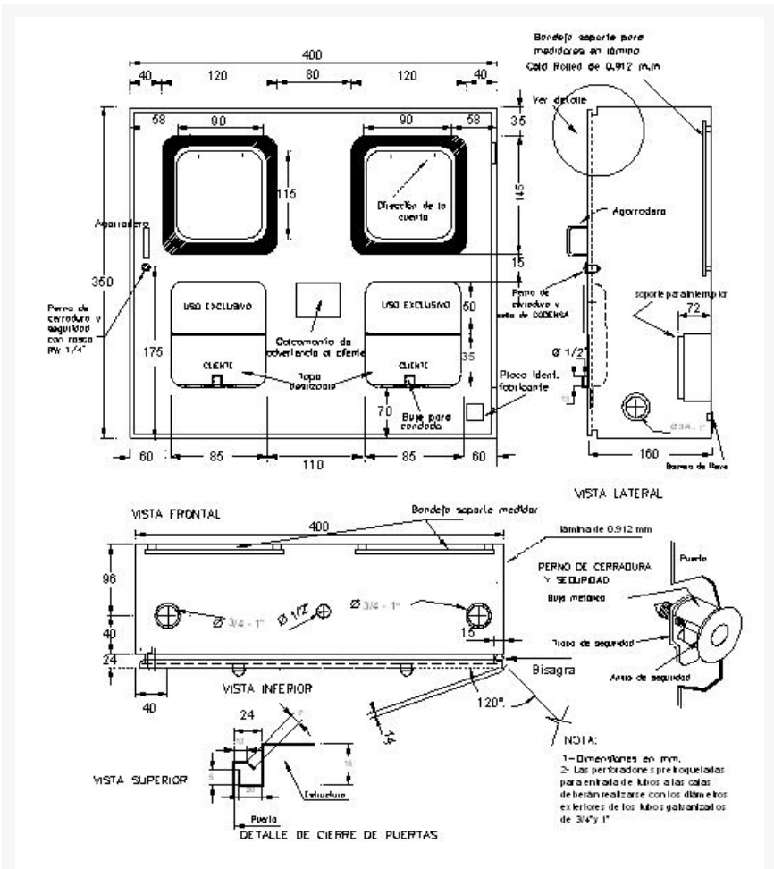
FIGURA 2: VISTA FRONTAL
