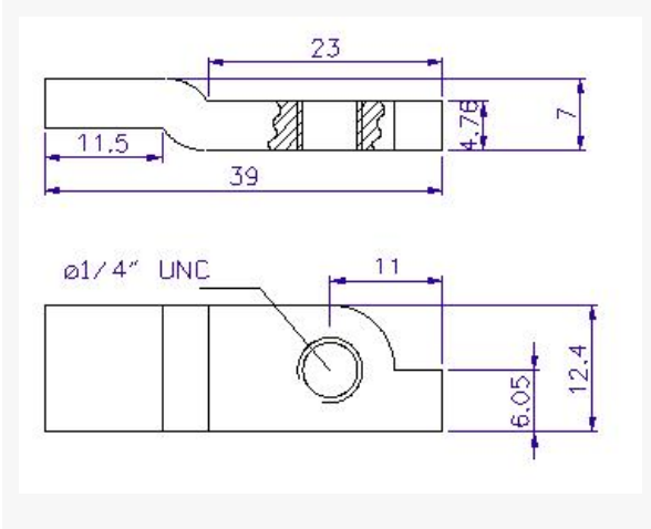
FIGURA 11. LLAVE PARA PERNO DEL SISTEMA DE SEGURIDAD
